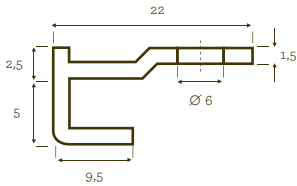
Profil de départ Edge profile Type F
