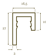
Profil de départ Edge profile Type CRP716
