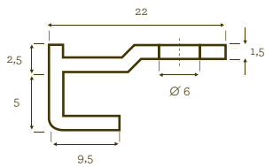
Profil de départ Edge profile Type F
